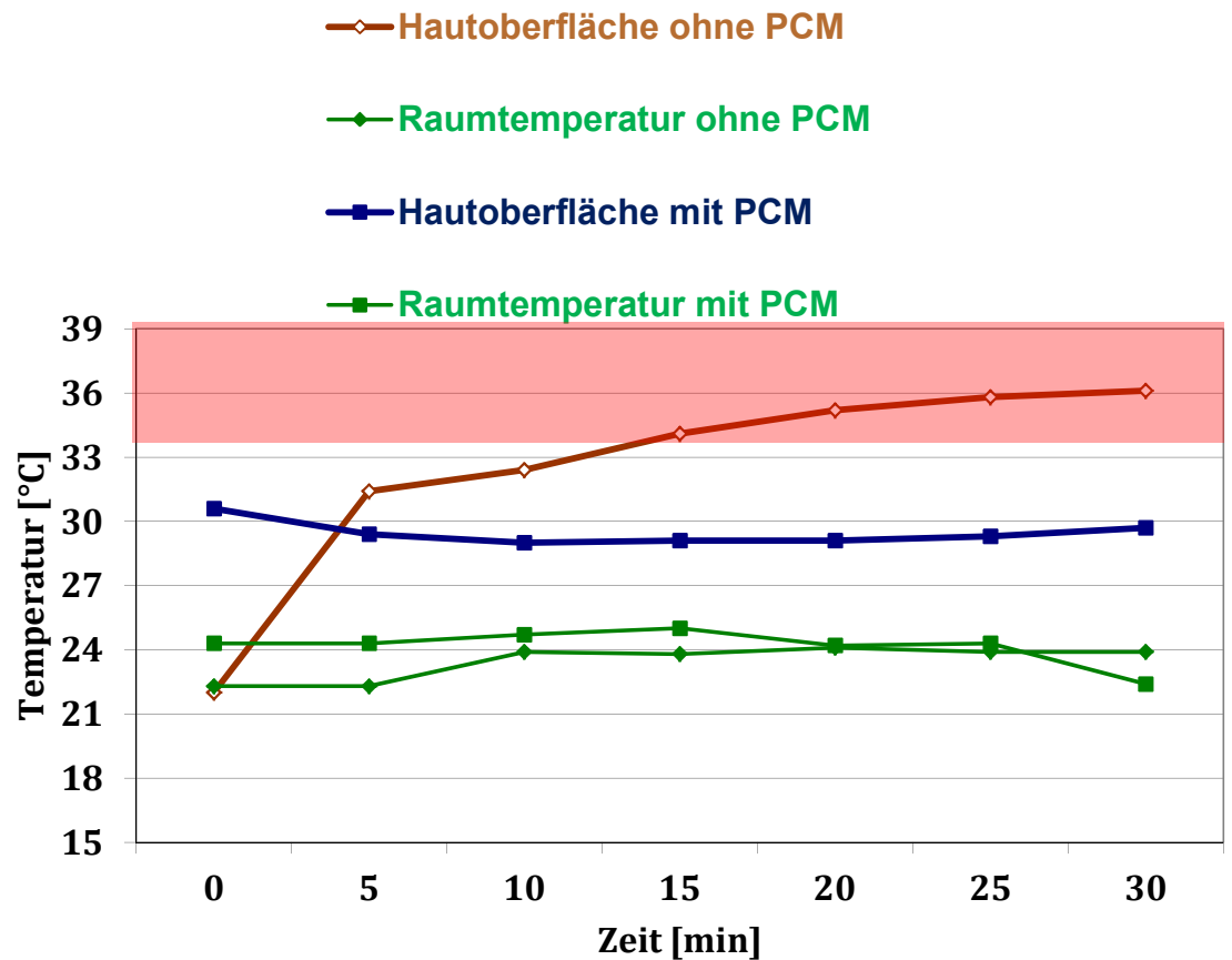
Temperaturaufzeichnung Prothese mit und ohne PCM-Einlage
